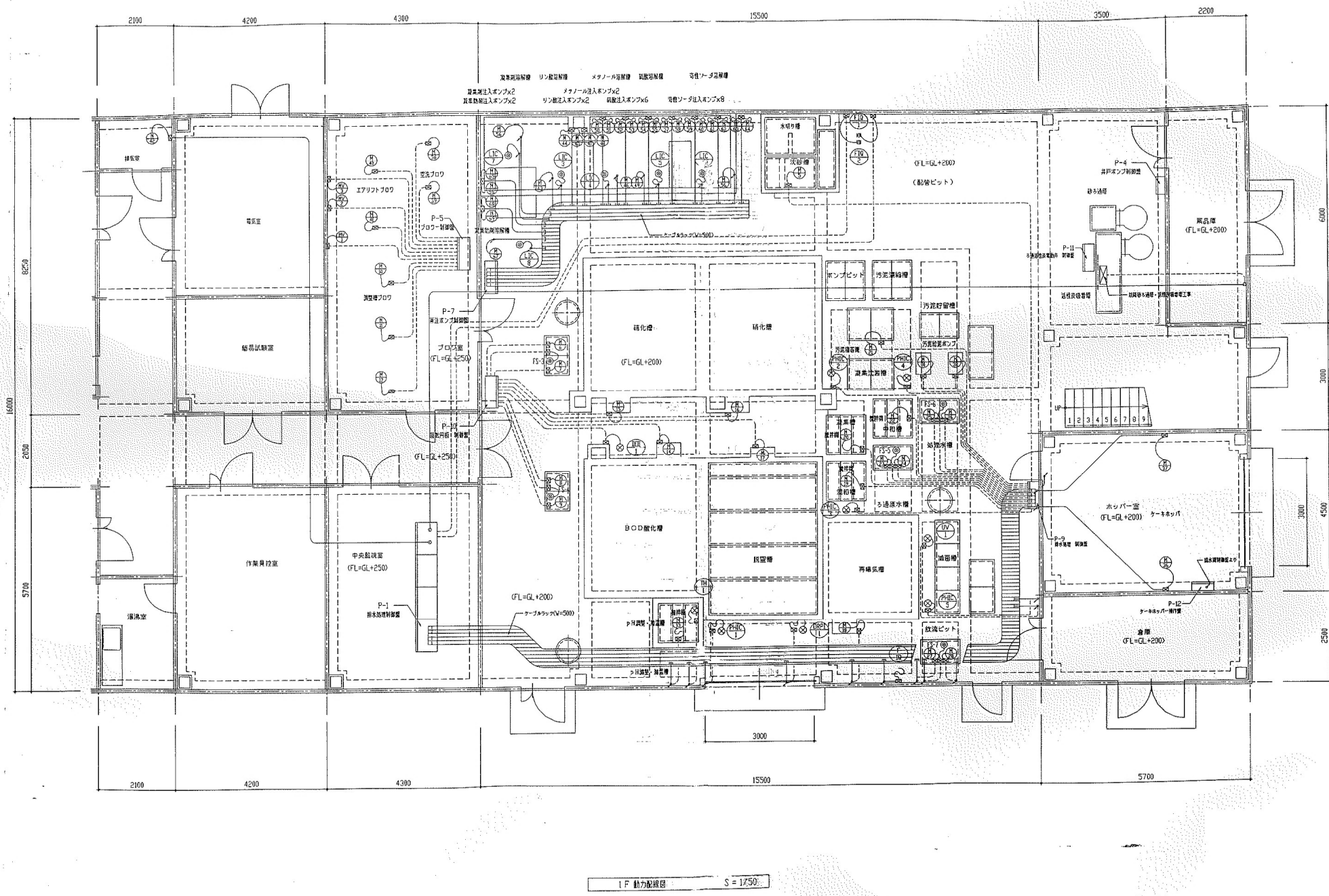
大崎広域一般廃棄物最終処分場 図面
